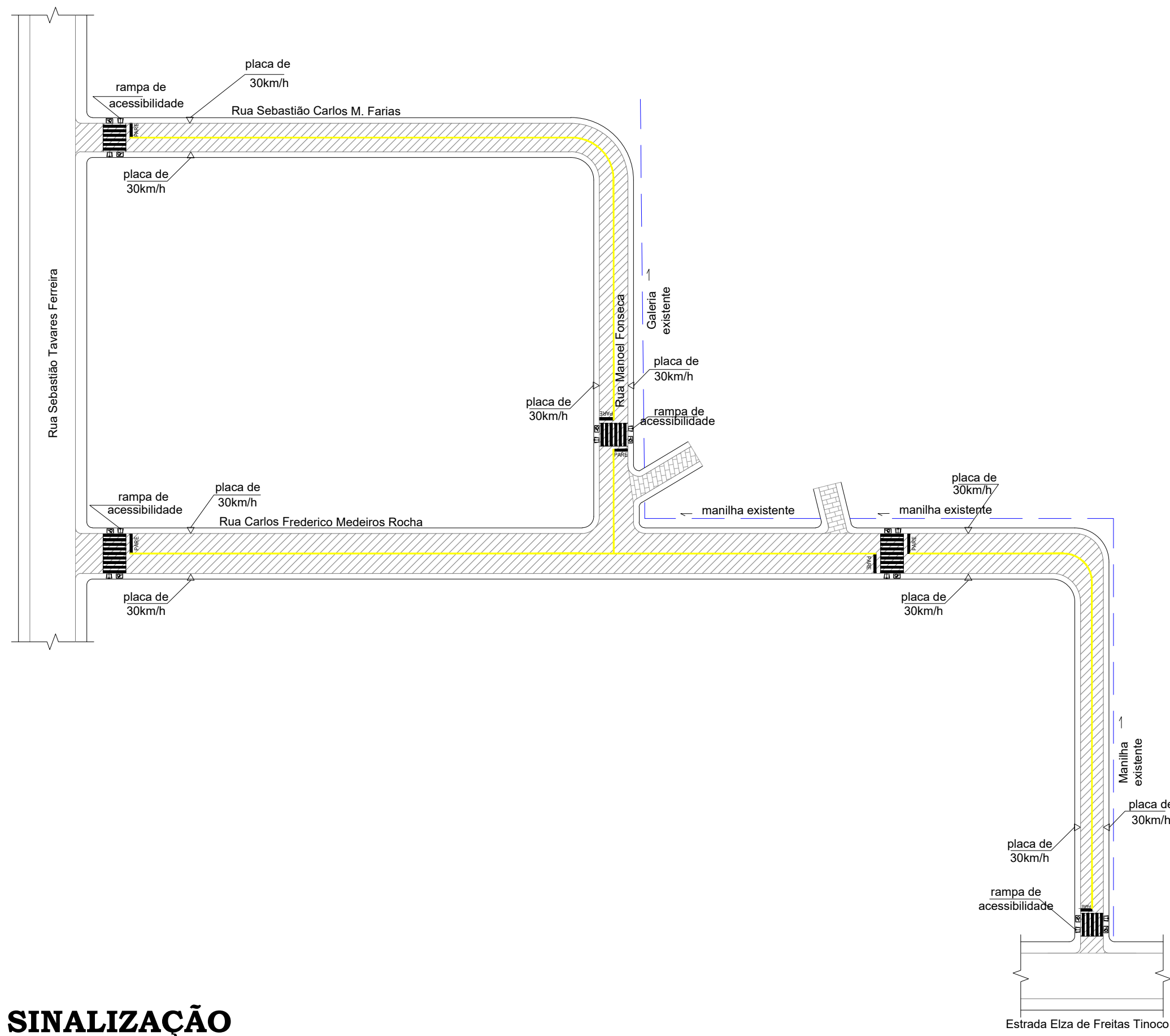
PROJETO SINALIZAÇÃO Escala: 1:750
