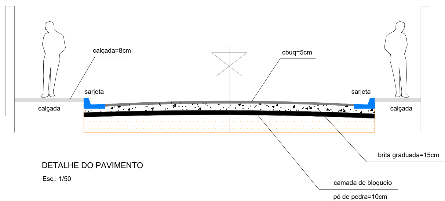
DETALHE DO PAVIMENTO Esc.: 1/50
